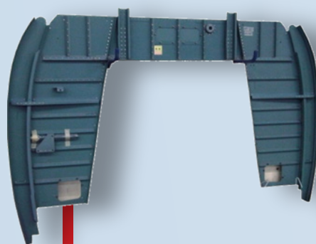
Cadre Airbus Helicopters
