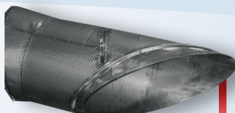
Carter Diffuseur Réacteur M53 Mirage 2000
