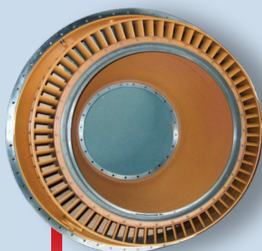
Carter Diffuseur Réacteur M53 Mirage 2000
